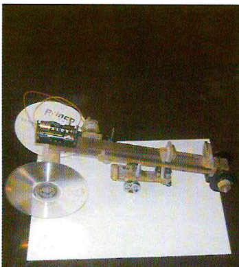
Figura 5. Prototipo No. 2. "vehículo" impulsado por fuerzas de atracción y repulsión magnética.
