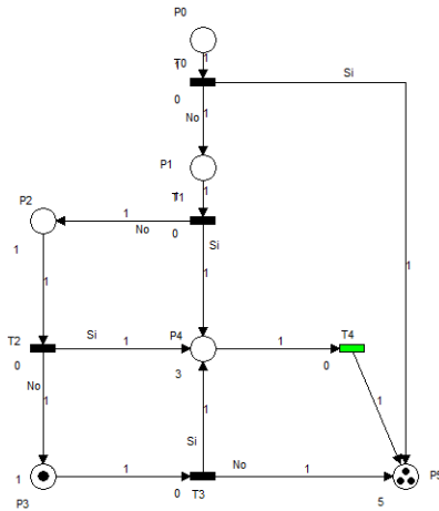
Figura 6: Ruta 1 de simulación
