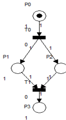
Figura 8: Modelado en RdP, Mejora del módulo de matriculación SGA UNEMI
