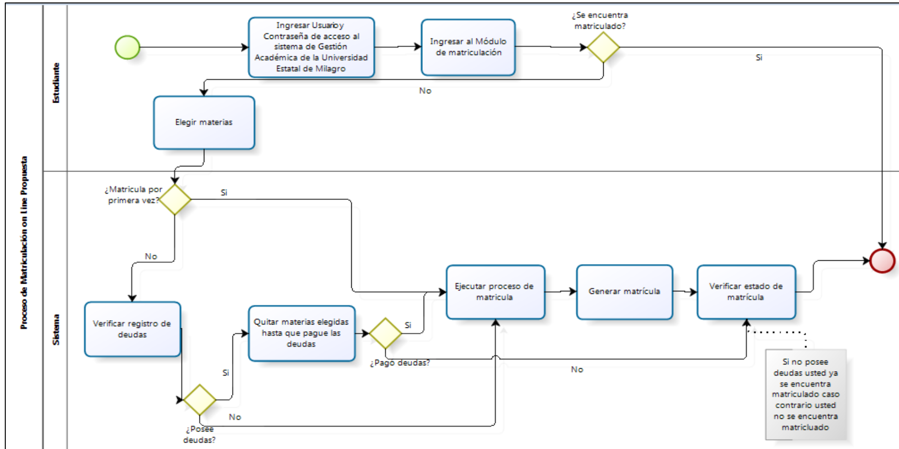
Figura 2: Modelado del Proceso del módulo de matriculación del SGA de la Universidad Estatal de Milagro
