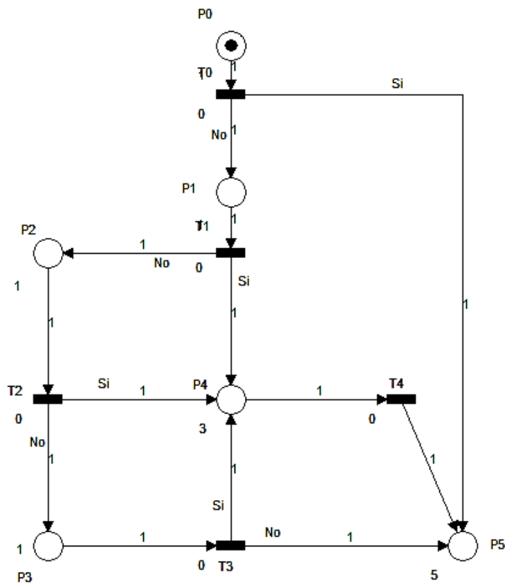
Figura 3: Modelado en RdP, módulo de matriculación SGA UNEMI
