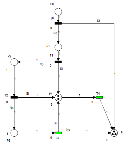
Figura 7: Ruta 2 de simulación
