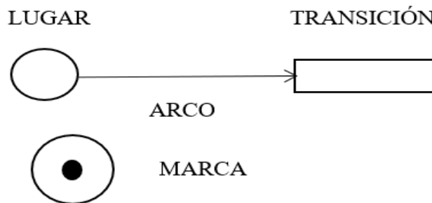
Figura 1: Identificación de componentes en una red de Petri
