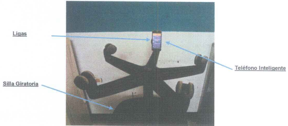
Ilustración 2. Grafica Montaje del Movimiento Circular Uniforme
