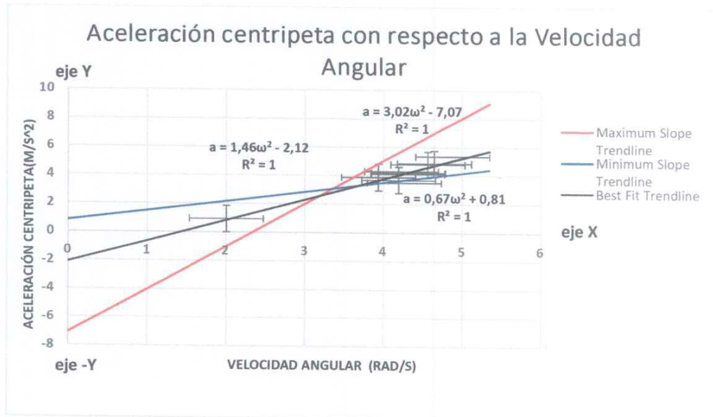
Ilustración 4: Grafica de Aceleración Centrípeta vs Velocidad Angular
