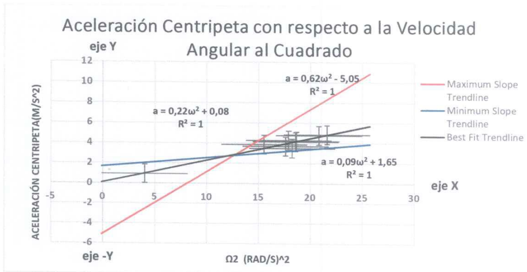
Ilustración 5: Gráfica de Aceleración Centrípeta vs Velocidad Angular al cuadrado
