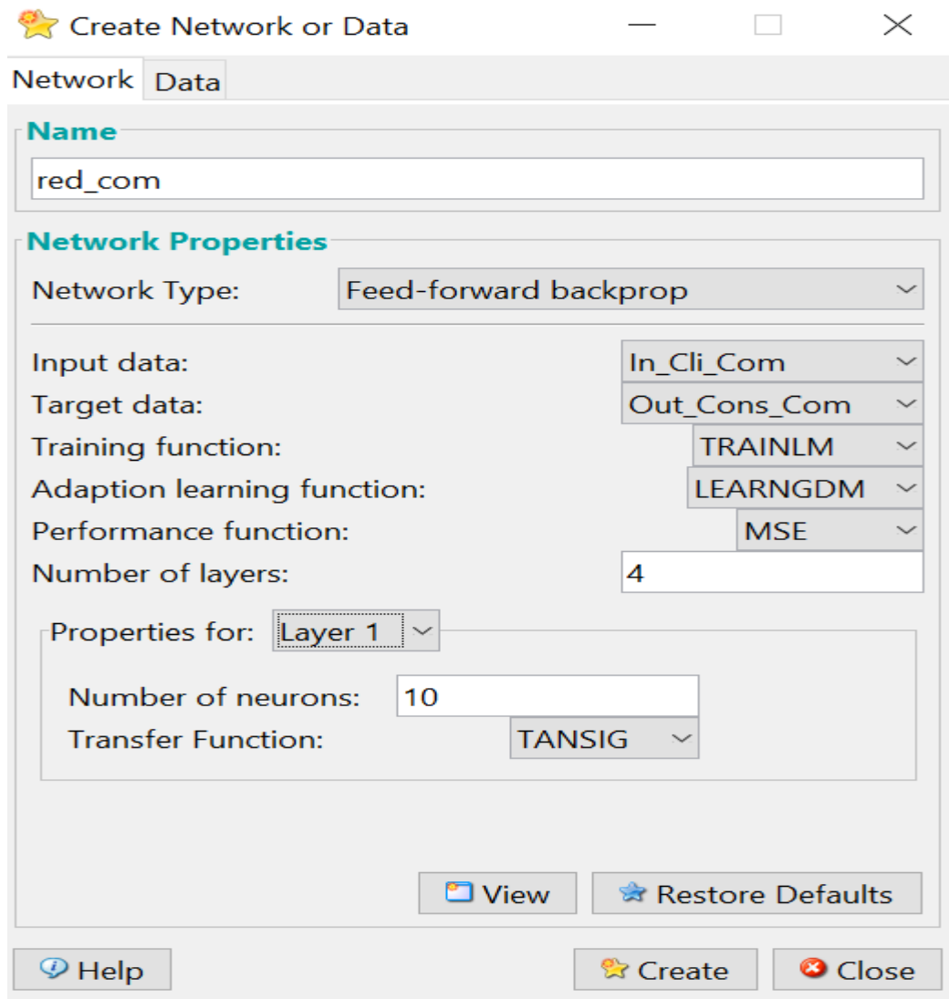
Figura 17. Creación de la red neuronal-Cliente Comerciales Fuente: Elaboración propia
