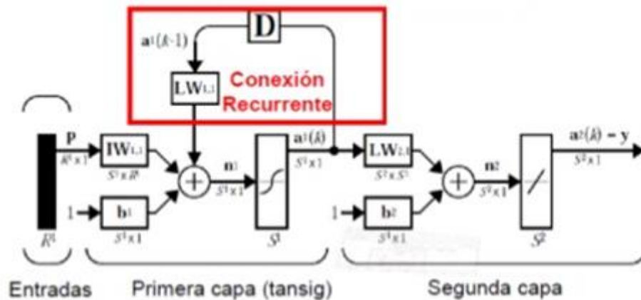
Figura 6. Redes Neuronales Recurrentes
