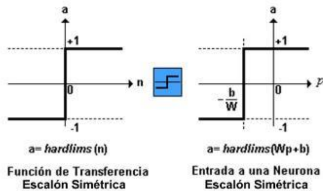
Figura 11. Modificación de Hardlim
