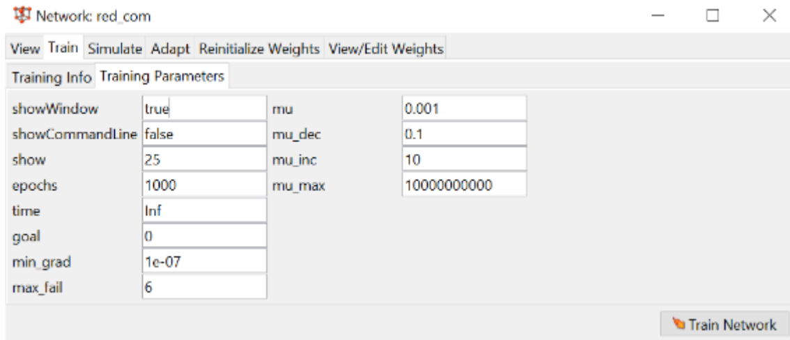
Figura 21. Parámetros de Entrenamiento Fuente: Elaboración Propia
