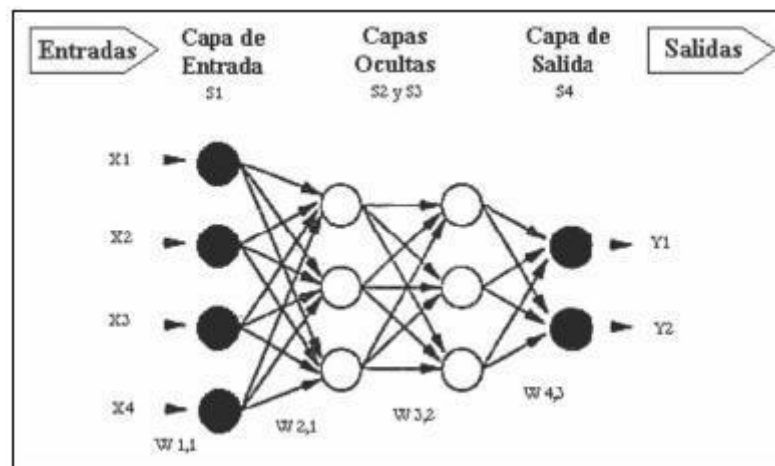
Figura 4. Red Multicapa
