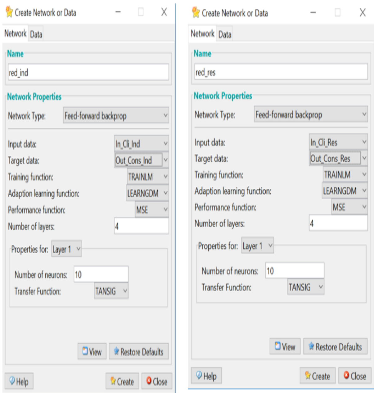
Figura 18. Creación de la red neuronal Clientes Industriales y Residenciales. Fuente: Elaboración propia
