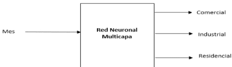
Figura 15. Red Neuronal usada para identificar un sistema
