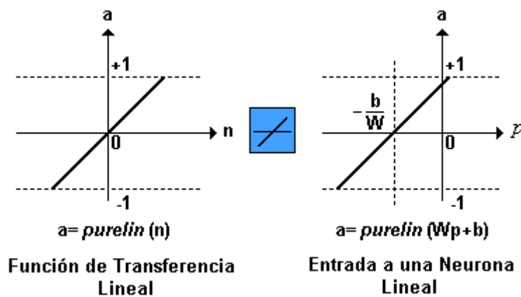
Figura 12. Función Purelin
