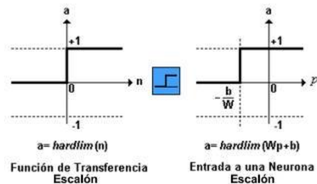
Figura 10. Función Hardlim
