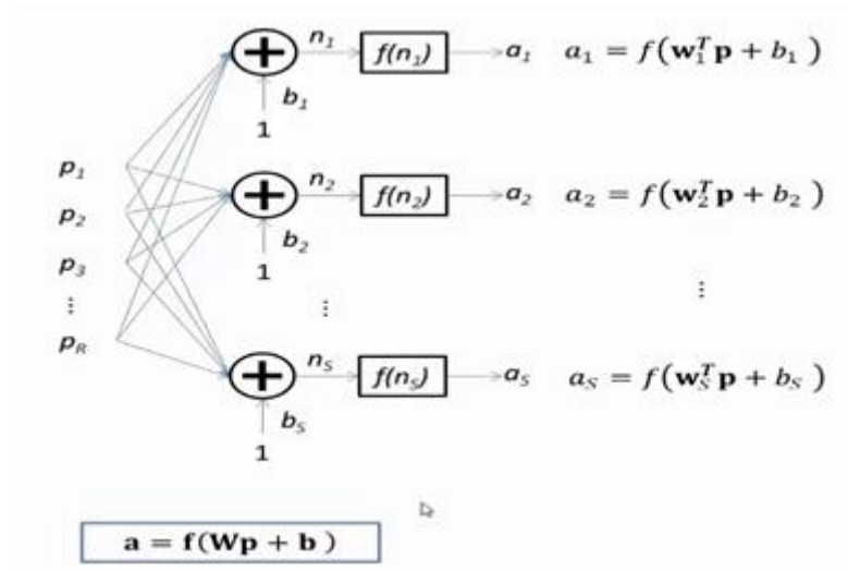
Figura 3. Red Monocapa
