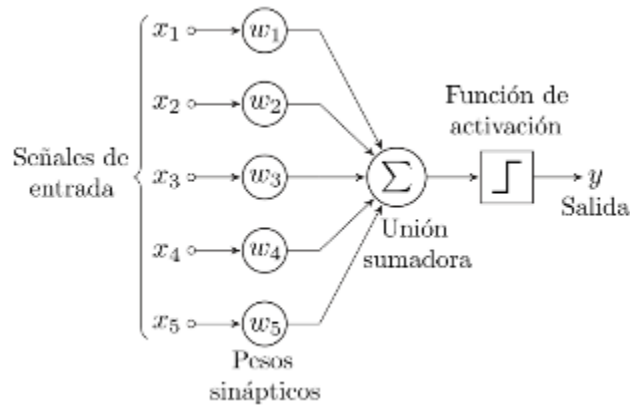
Figura 7. Red Perceptrón
