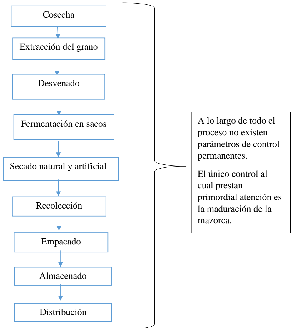
Cuadro #. 1 Flujograma de procesos actuales en Zhucay. Fuente: del autor
