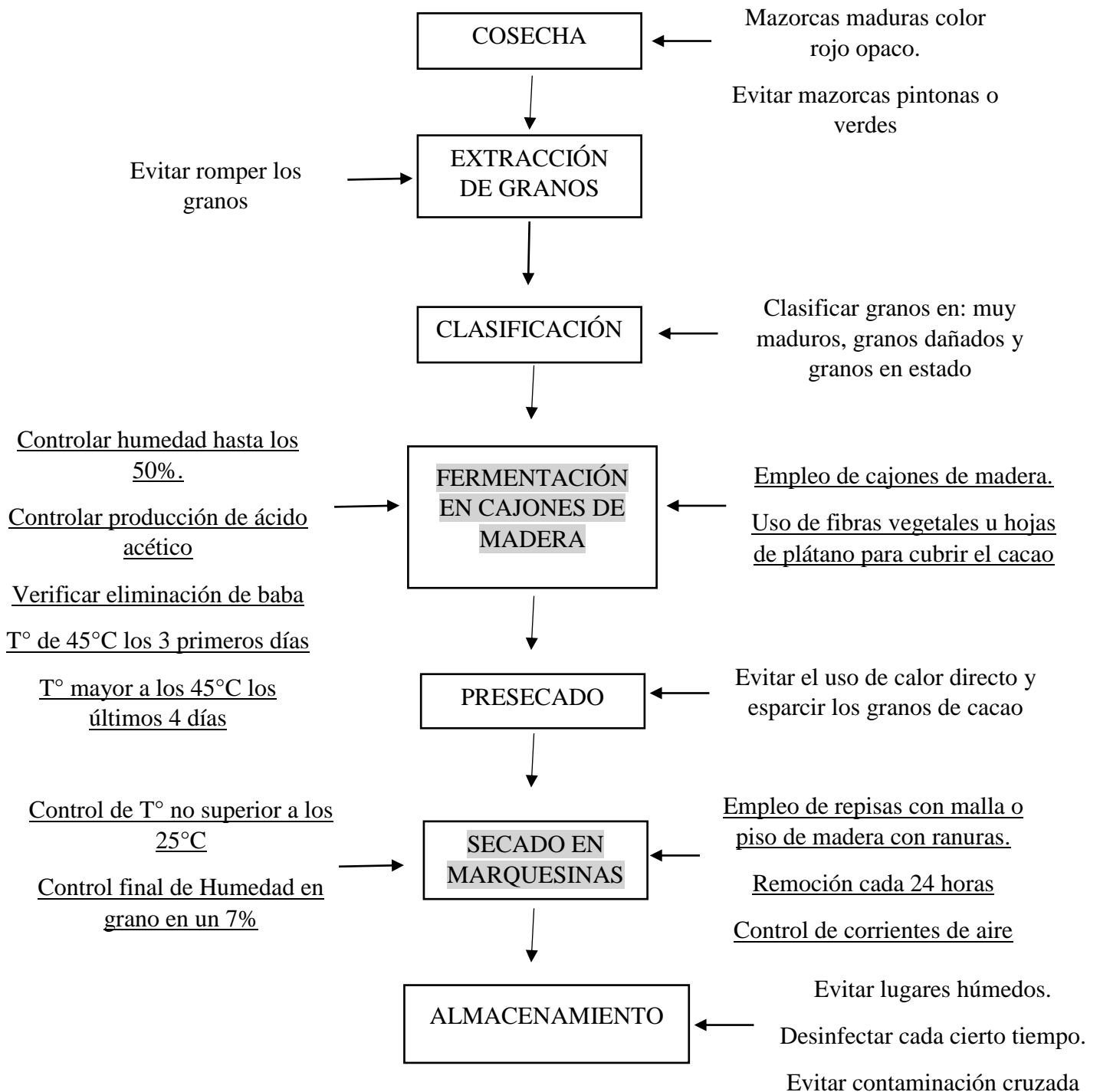
Cuadro #3. Diagrama de flujo con Puntos Críticos de Control. Fuente: del autor
