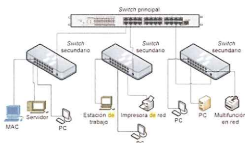
Figura 4 Conexión de red Ethernet. Esquema general de conexiones de equipos
